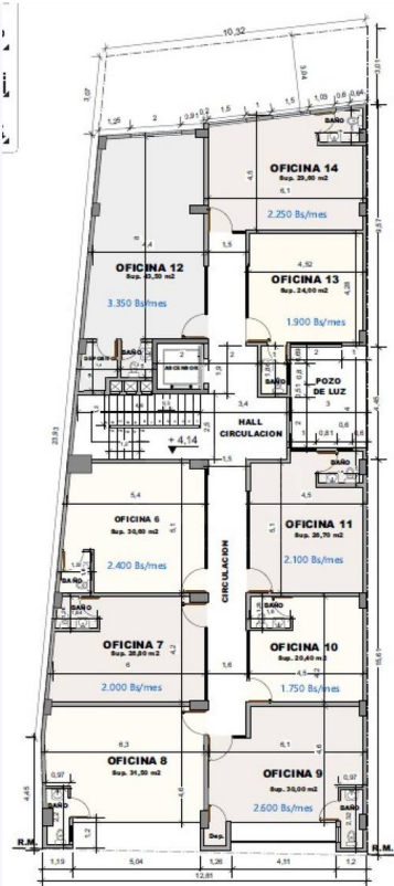
1er PISO
